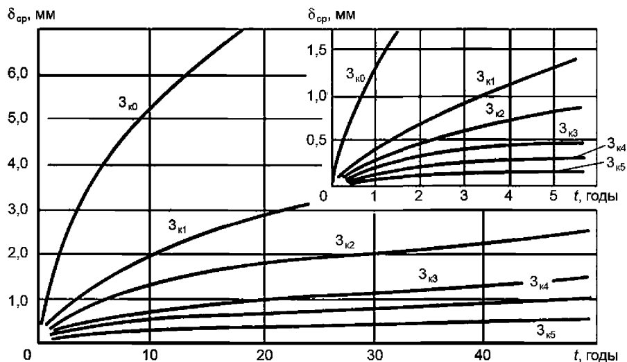
Рисунок 1 — Зависимость глубины коррозии стальных заземлителей \delta_{\text{op}} от времени для различных коррозионных зон
